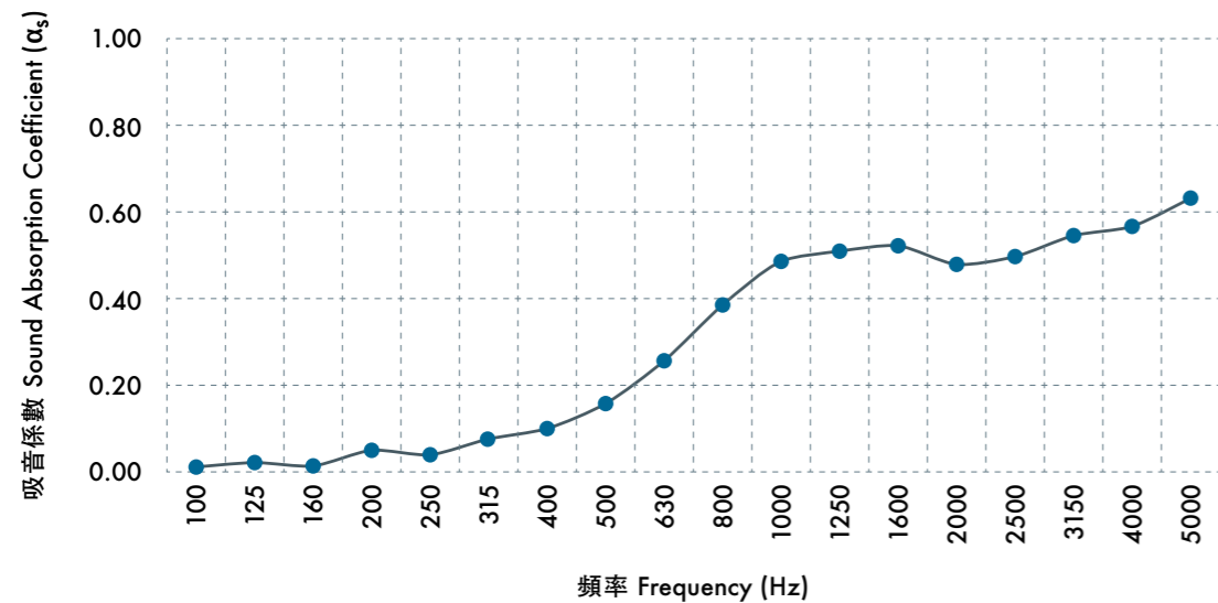
有機軟木塊吸音係數圖
